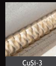
CuSi-3
