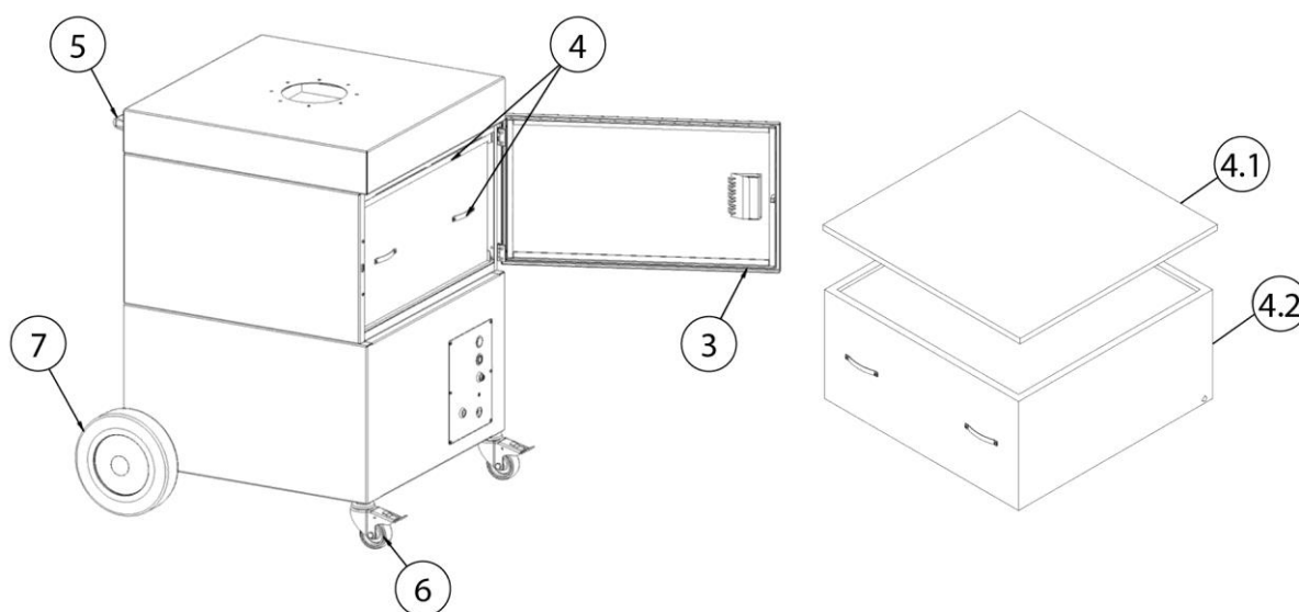
Afb. 31: Montage
