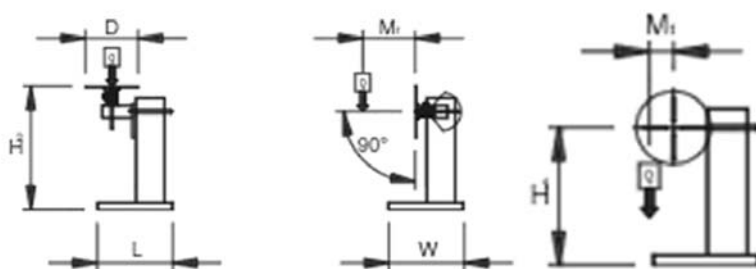
Verticaal draagvermogen tov lengte van het werkstuk (symmetrisch)
