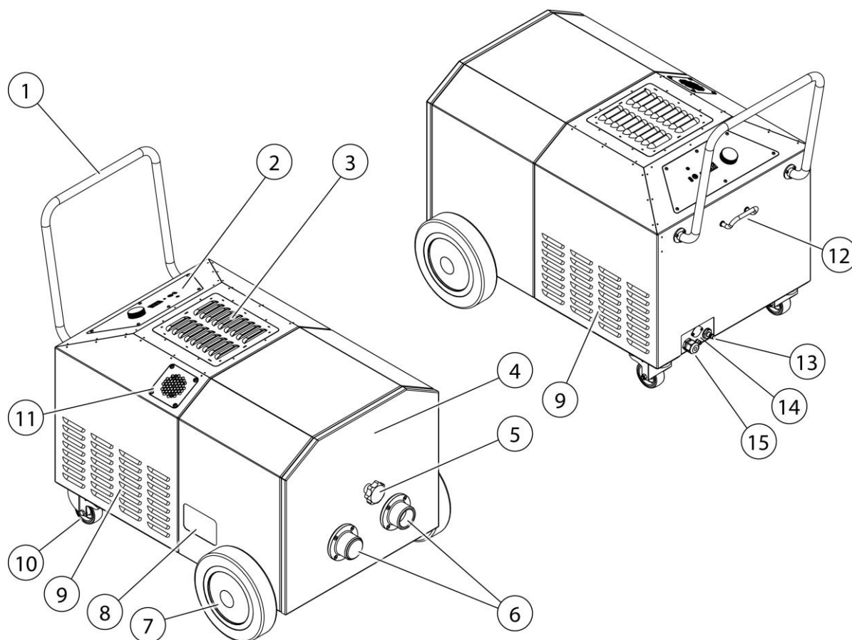
Afb. 52: Functiebeschrijving – product
