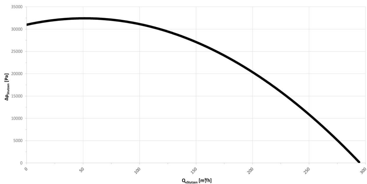
Afb. 67: Karakteristiek
