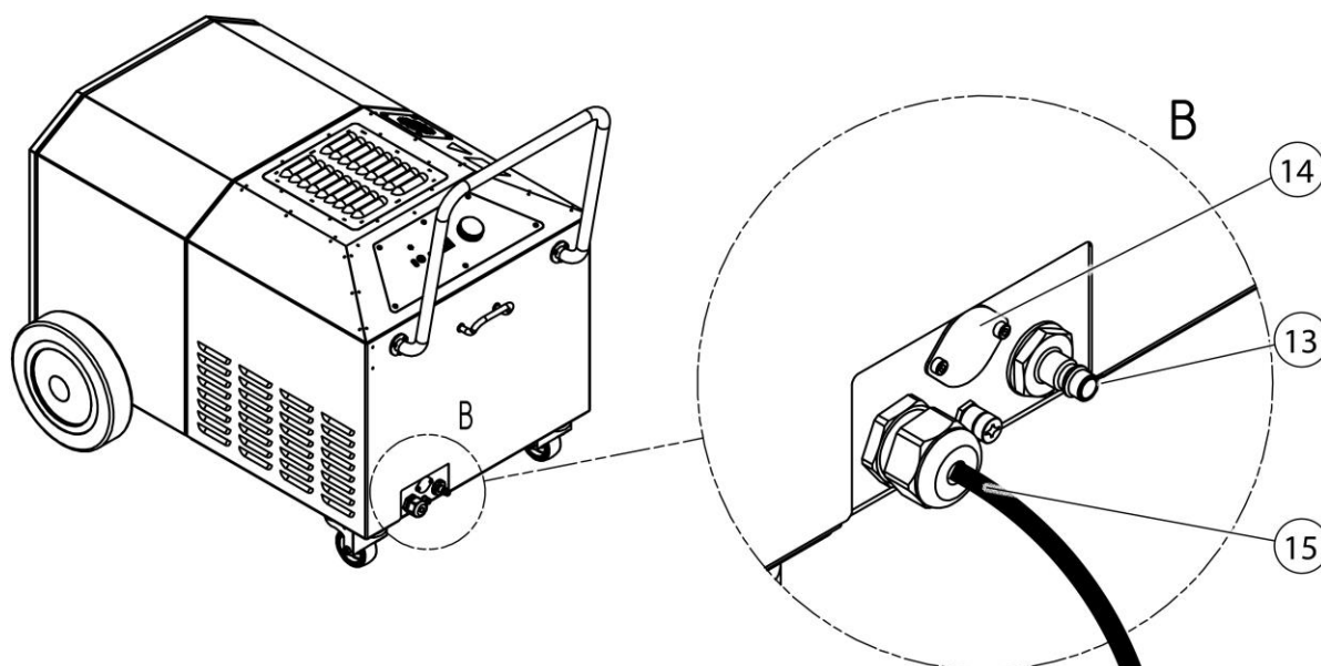
Afb. 53: Aansluitingen
