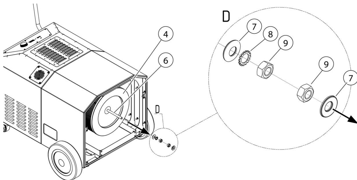
Afb. 61: Hoofdfilter demonteren
